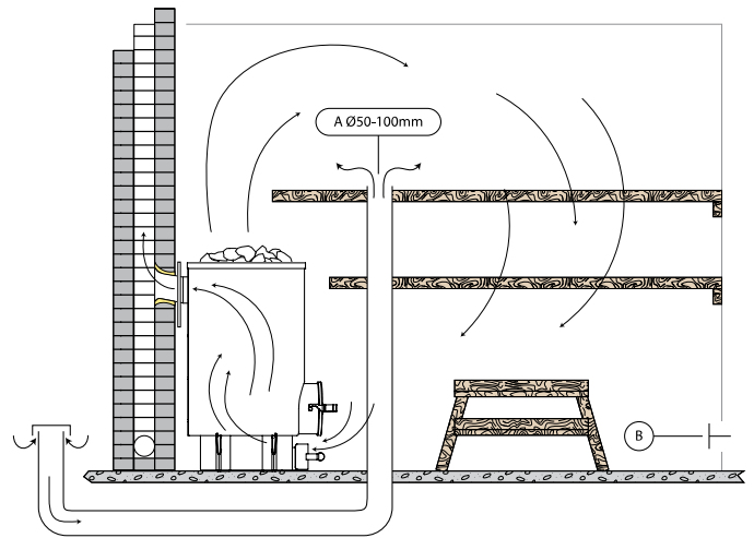
Kuva 4: Koneellinen ilmanvaihto Bild 4: Maskinell ventilation Picture 4: Mechanical ventilation
