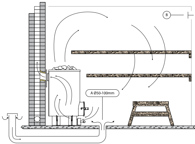
Kuva 3: Painovoimainen ilmanvaihto Bild 3: Självdagsventilation Picture 3: Gravity ventilation
